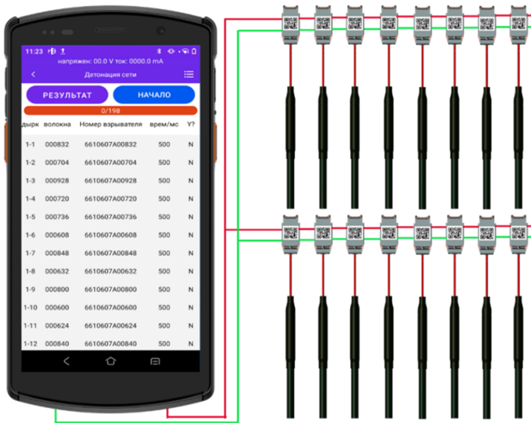
应用接线示意图
